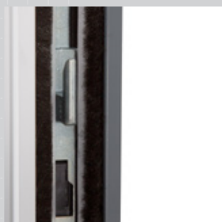
Crochets métalliques pris directement dans le profilé Crémone 1 à 4 pt selon hauteur
